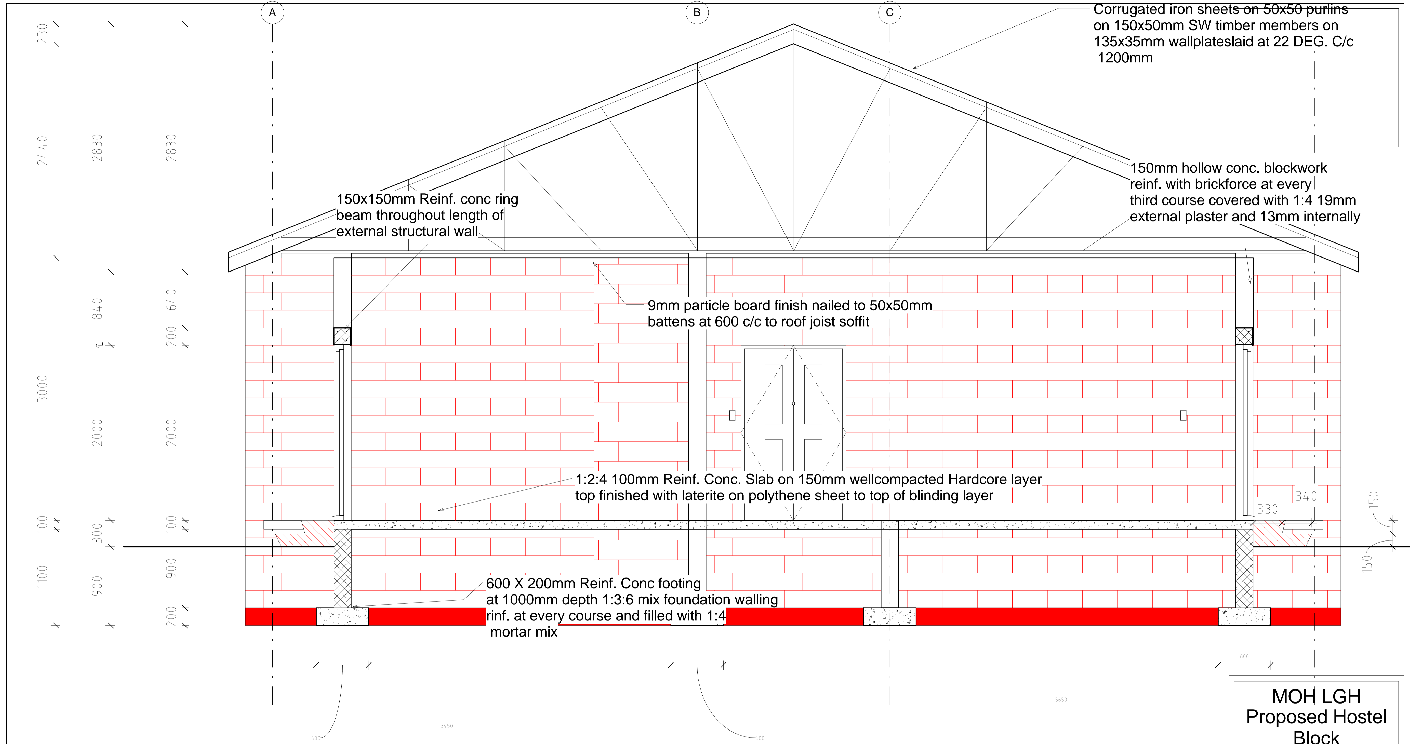
1 Section 1 1 : 20
